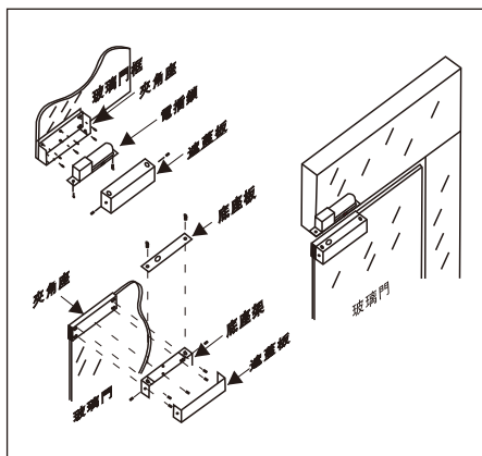
電插鎖支架安裝效果
