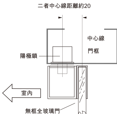
BBK-601剖视图
